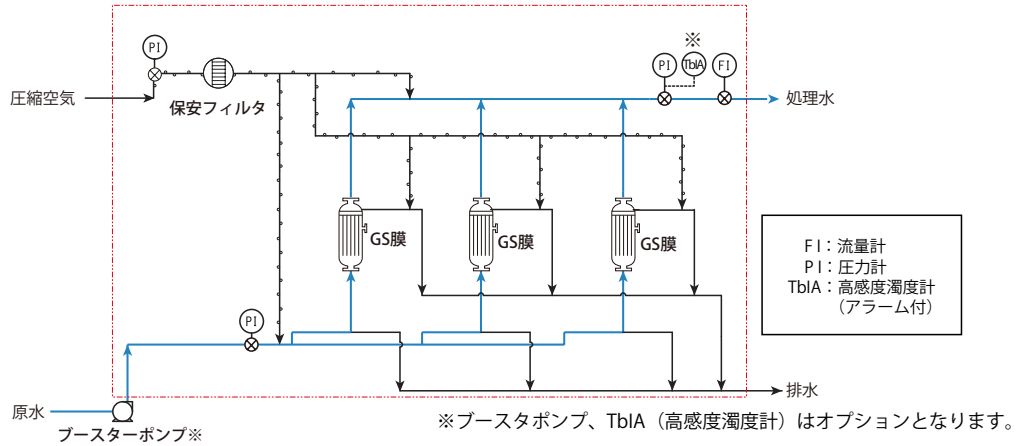
膜式前処理装置 PF-GS-V 型 (フロー図)
