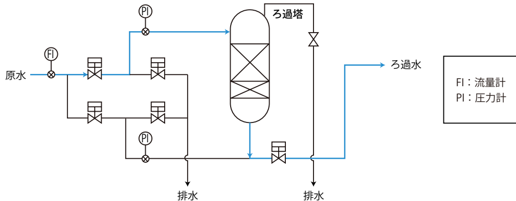
活性炭ろ過器 KA-A型(フロー図)
