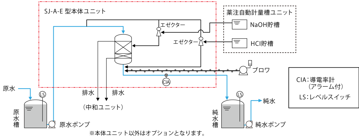
混床式自動純水装置 SJ-A-E型 (フロー図)
