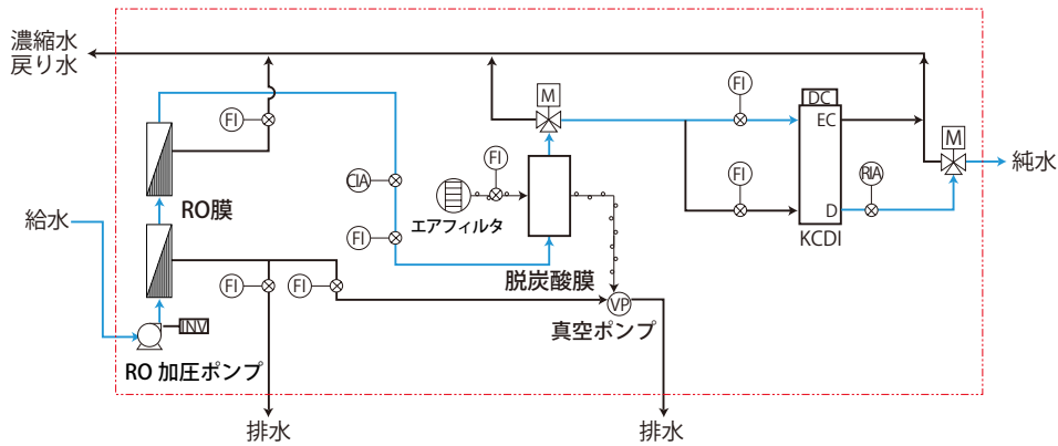
連続再生式純水装置 ピュアエース R-PA-W 型 (フロー図)
